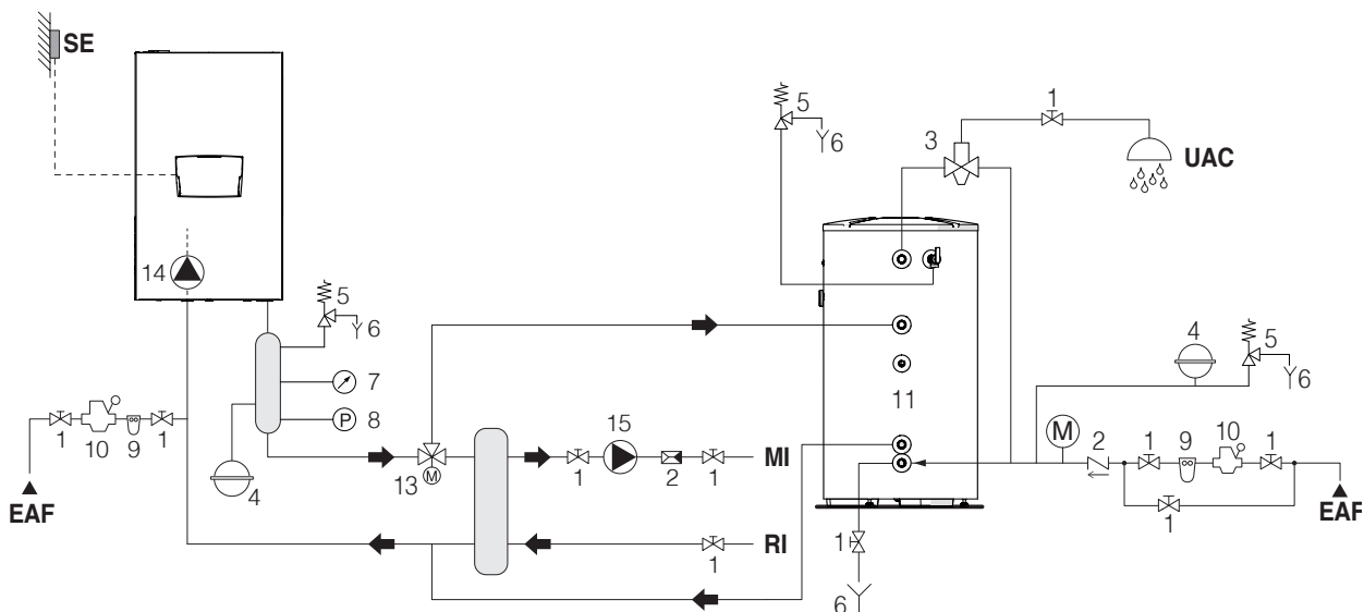
Schéma 5: obvod s tepelným modulom spojený s vykurovacím rozvadom a s nádržou TUV prostredníctvom separátora
