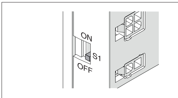
Configuración del interruptor S1=OFF
