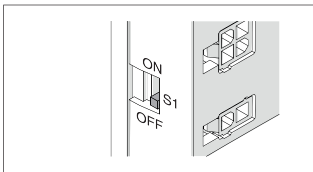
Podešavanje prekidača S1=OFF
