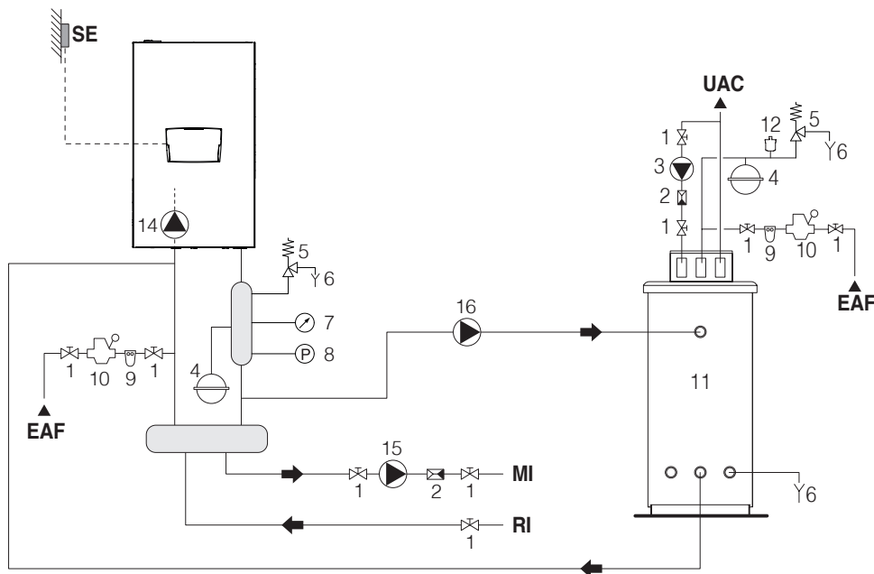
Esquema 4: circuito com módulo térmico ligado ao reservatório de AQS e à instalação de aquecimento através de um separador
