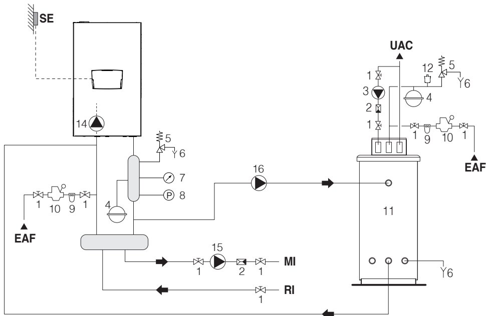
Diagrama 4: circuit cu modul termic conectat la rezervor ACM și la instalație de încălzire prin intermediul unui separator
