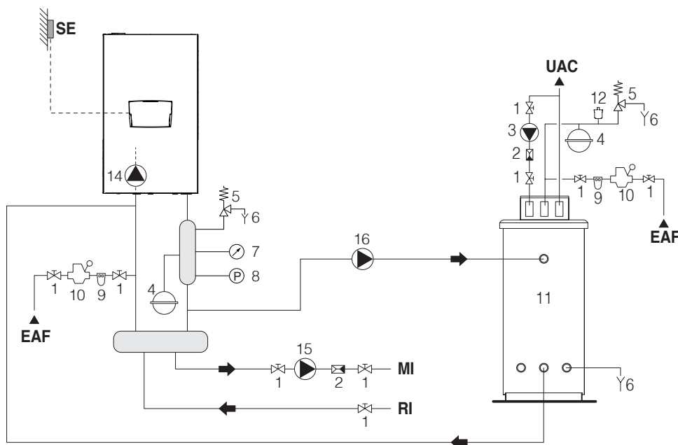
Schema 4: krogotok, pri katerem je toplotni modul z rezervoarjem TSV in ogrevalnim sistemom povezan prek ločevalnika
