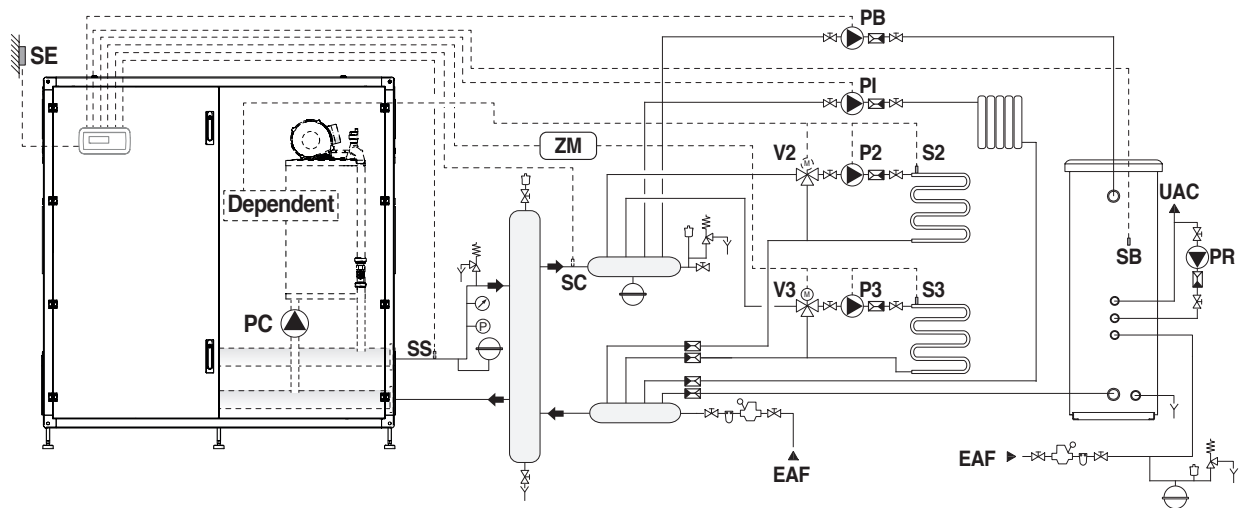
Šema 2: Krug sa termičkim modulima koji imaju vlastitu cirkulacionu pumpu i spojeni su u kaskadu. Upotreba sonde sekundarnog kruga.
