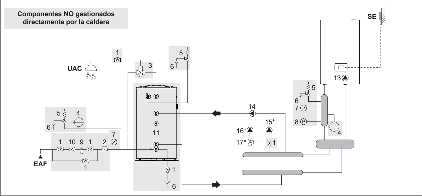
Esquema 4: circuito con caldera conectada con depósito de A.C.S. y con instalación de calentamiento mediante separador
