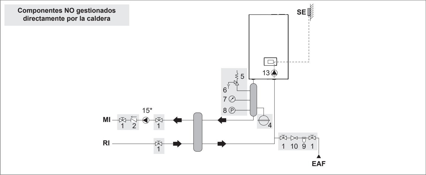
Esquema 4: circuito con caldera conectada con depósito de A.C.S. y con instalación de calentamiento mediante separador
