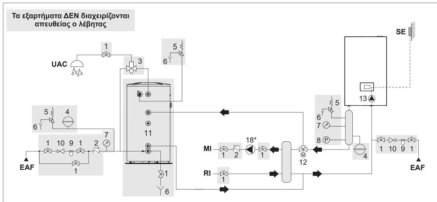
Διάταξη 5: κύκλωμα με λέβητα συνδεδεμένο με το σύστημα θέρμανσης και τη δεξαμενή ZNX μέσω υδραυλικού διαχωριστή
