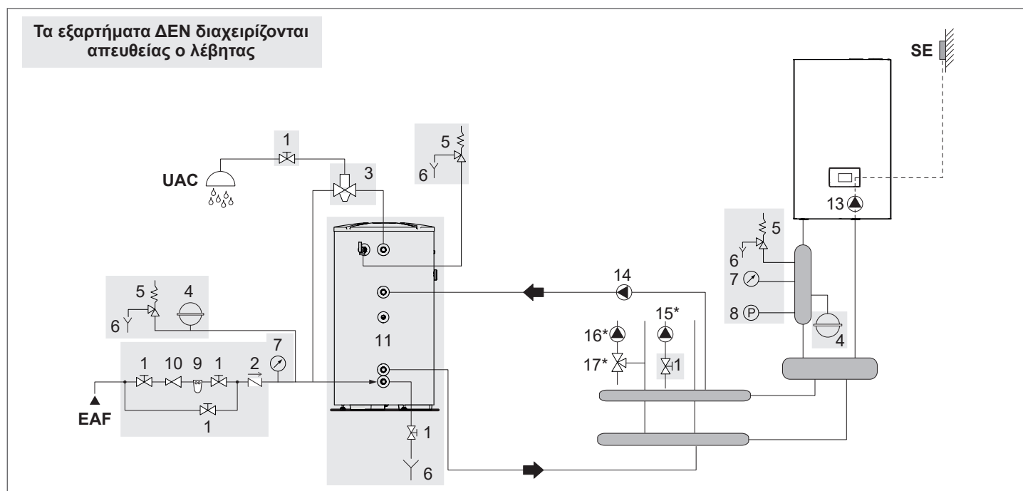
Διάταξη 4: κύκλωμα με λέβητα συνδεδεμένο με δεξαμενή ΖΝΧ και σύστημα θέρμανσης μέσω υδραυλικού διαχωριστή
