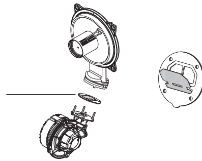
16 Clapet
