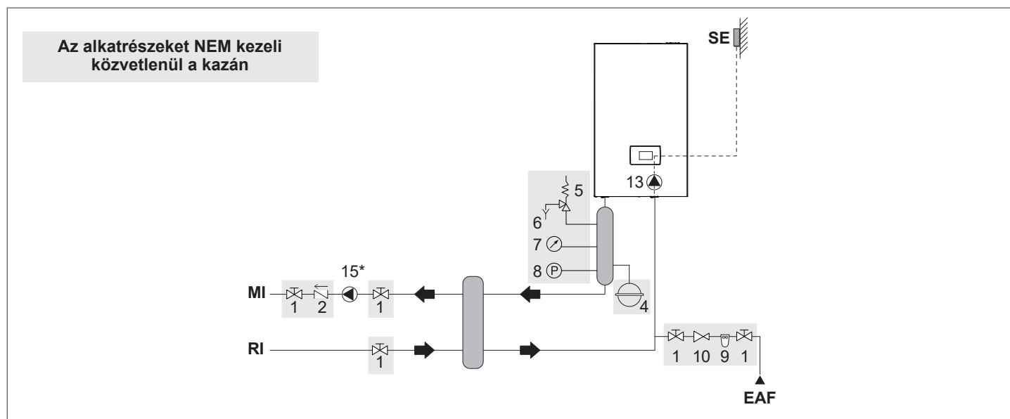
3 rajz: elválasztóval fűtési rendszerrel csatlakoztatott kazános kör
