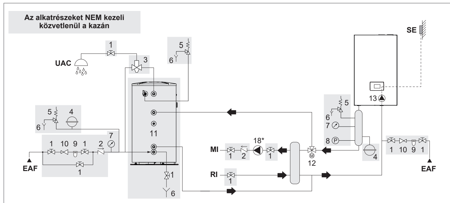
5 rajz: szétválasztóval HMV tartállyal és fűtőrendszerrel csatlakoztatott kazános kör
