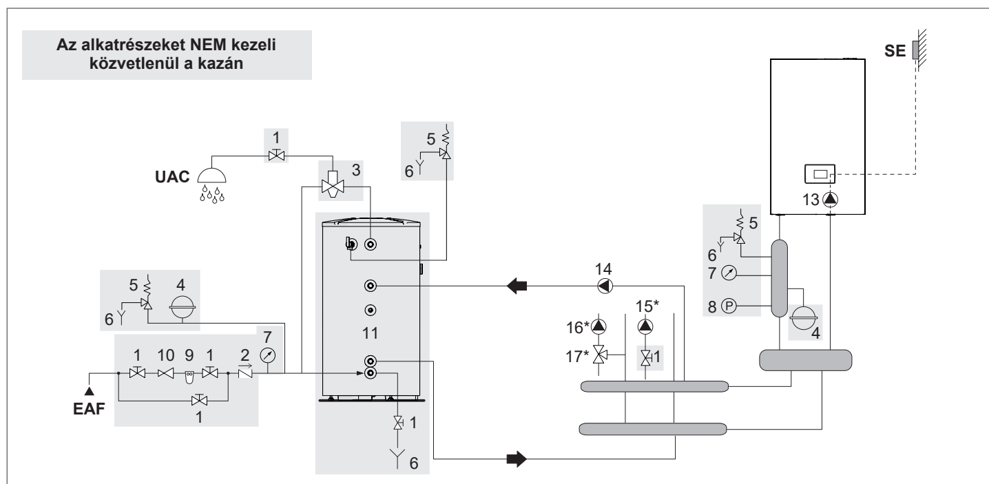
4 rajz: kör a használati meleg víz tartályhoz csatlakoztatott kazánnal és fűtési rendszerrel elválasztóval
