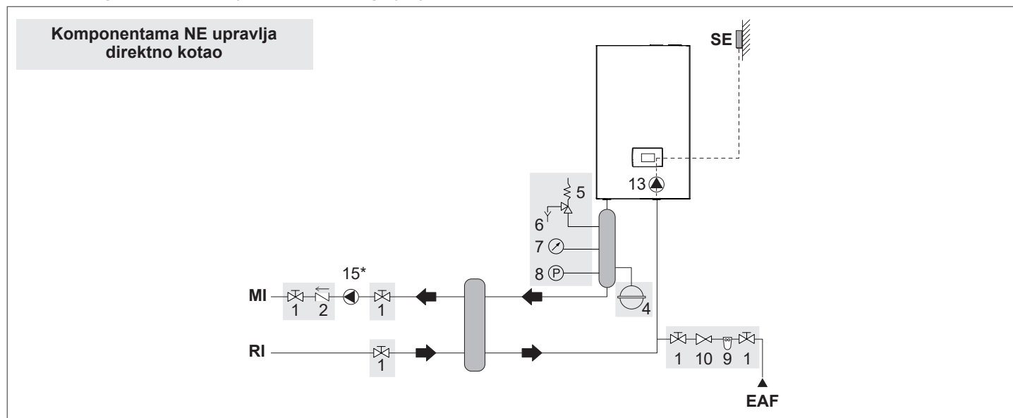
Šema 3: krug sa kotlom priključen na sistem grejanja pomoću hidrauličke skretnice
