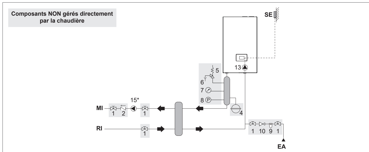
Schéma 4: circuit avec une chaudière connectée au réservoir d'ECS et au système de chauffage au moyen d'un séparateur.
