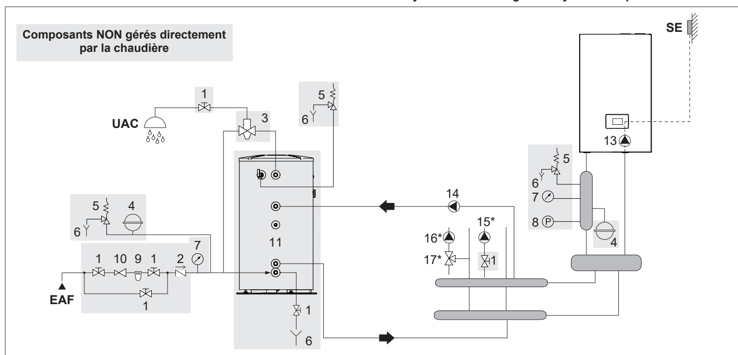
Schéma 4: circuit avec une chaudière connectée au réservoir d'ECS et au système de chauffage au moyen d'un séparateur.
