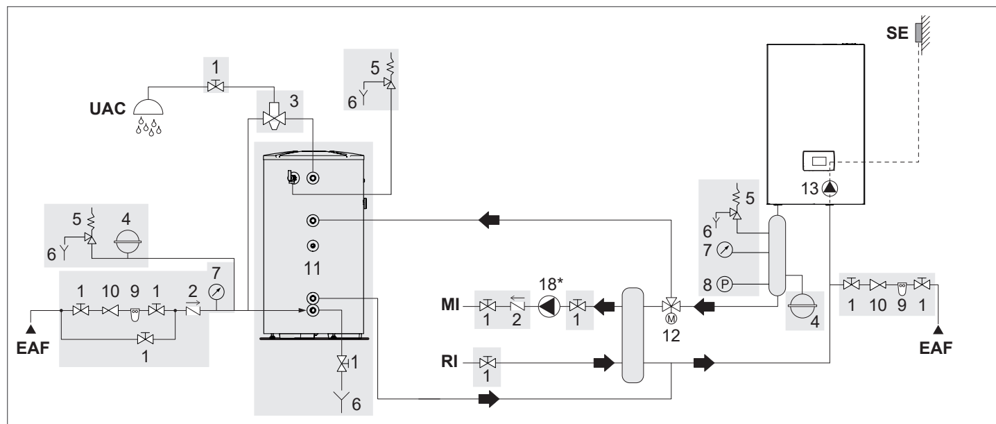
Schéma 5: circuit avec une chaudière connectée au système de chauffage et au réservoir d'ECS au moyen d'un séparateur.
