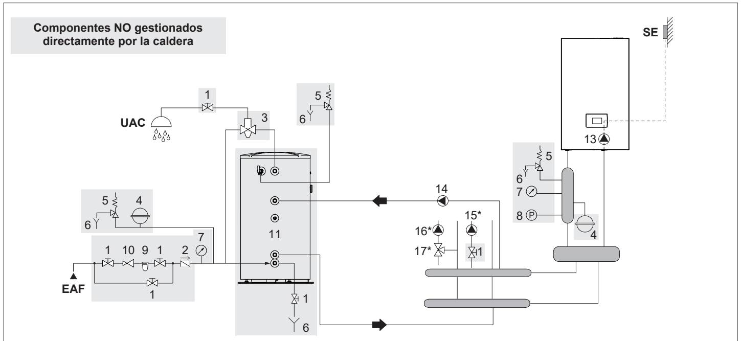
Esquema 4: circuito con caldera conectada con depósito de A.C.S. y con instalación de calentamiento mediante separador
