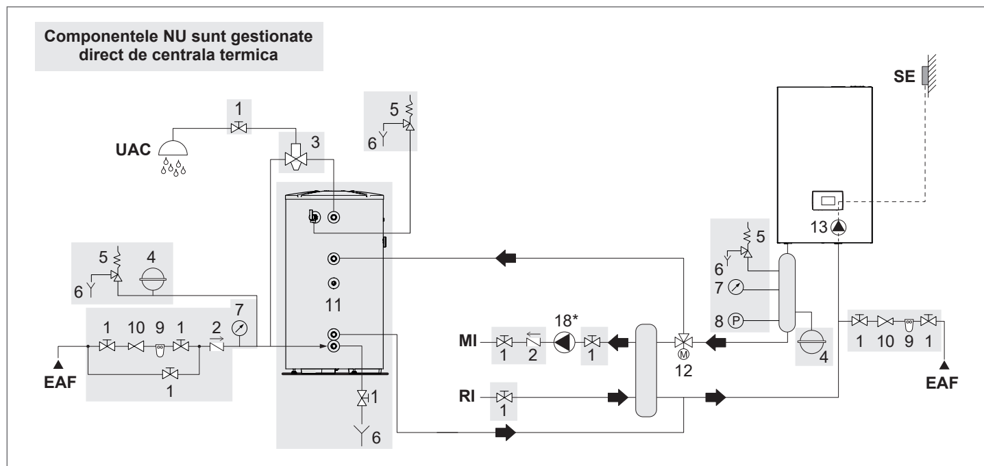
Schema 5: circuit cu centrală conectată la instalația de încălzire și rezervorul ACM prin intermediul unui separator hidraulic
