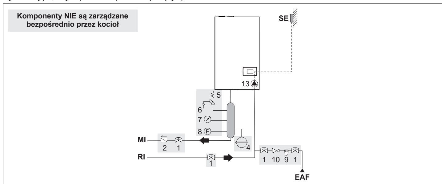
Schemat 2: obwód z kotłem podłączonym bezpośrednio do instalacji grzewczej i zbiornika c.w.u. (sprawdzić, czy ciśnienie tłoczenia pompy jest wystarczające, aby zapewnić odpowiedni przepływ)
