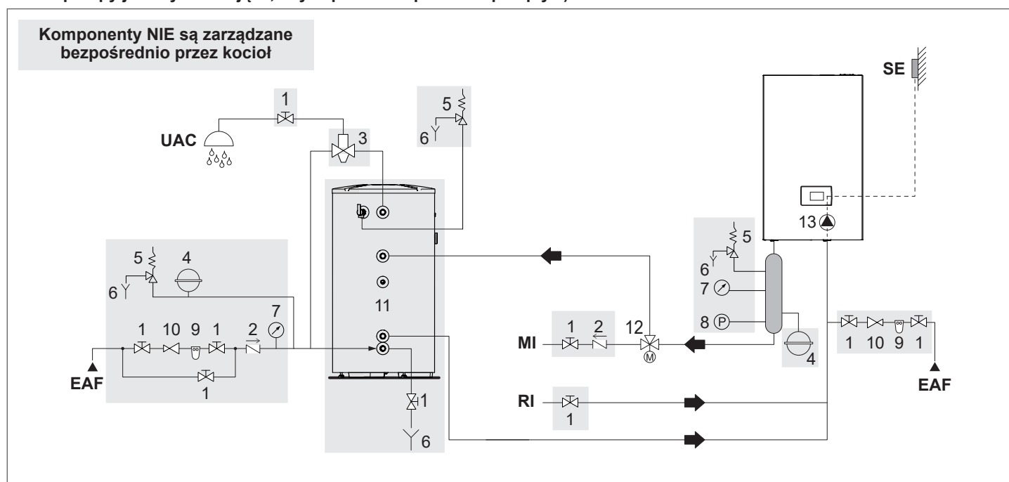
Schemat 2: obwód z kotłem podłączonym bezpośrednio do instalacji grzewczej i zbiornika c.w.u. (sprawdzić, czy ciśnienie tłoczenia pompy jest wystarczające, aby zapewnić odpowiedni przepływ)
