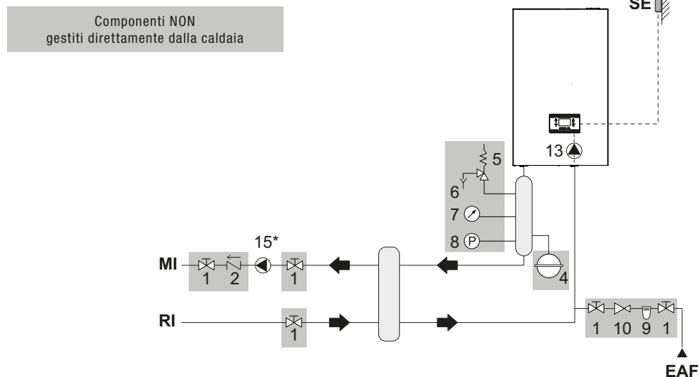
Schema 4: circuito con caldaia collegata con serbatoio A.C.S. e con impianto di riscaldamento tramite separatore.
