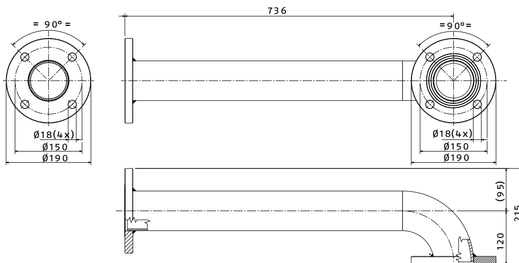
3" DN80 PN6
