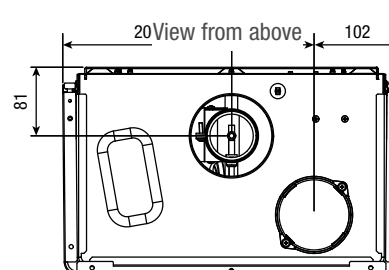
Vista dall'alto
