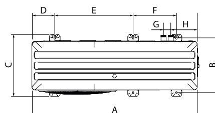
8/10/12/14/16 kW (dimensions en mm)
