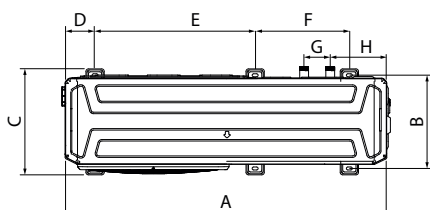
4/6 kW (dimensions en mm)
