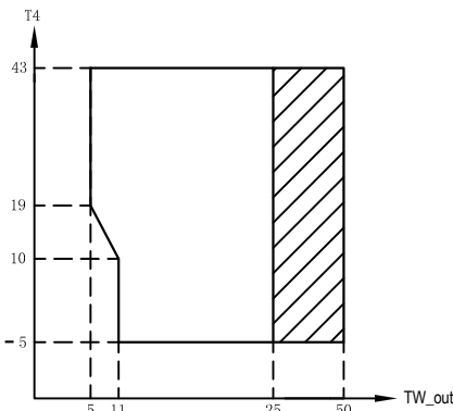
Plage de fonctionnement par pompe à chaleur avec limitation et protection possibles.
