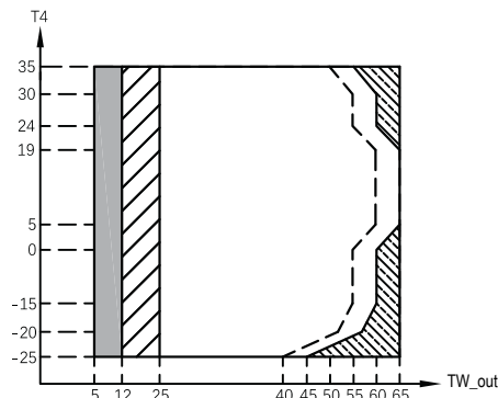
Si le réglage IBH/AHS est valide, seul IBH/AHS s'allume. Si le réglage IBH/AHS n'est pas valide, seul la pompe à chaleur s'allume. Il peut y avoir des cas de limitation et de protection pendant le fonctionnement de la pompe à chaleur. Plage de fonctionnement par pompe à chaleur avec limitation et protection possibles. La pompe à chaleur s'éteint, seul IBH/AHS s'allume. --- Ligne de température maximale d'entrée d'eau pour le fonctionnement de la pompe à chaleur.
