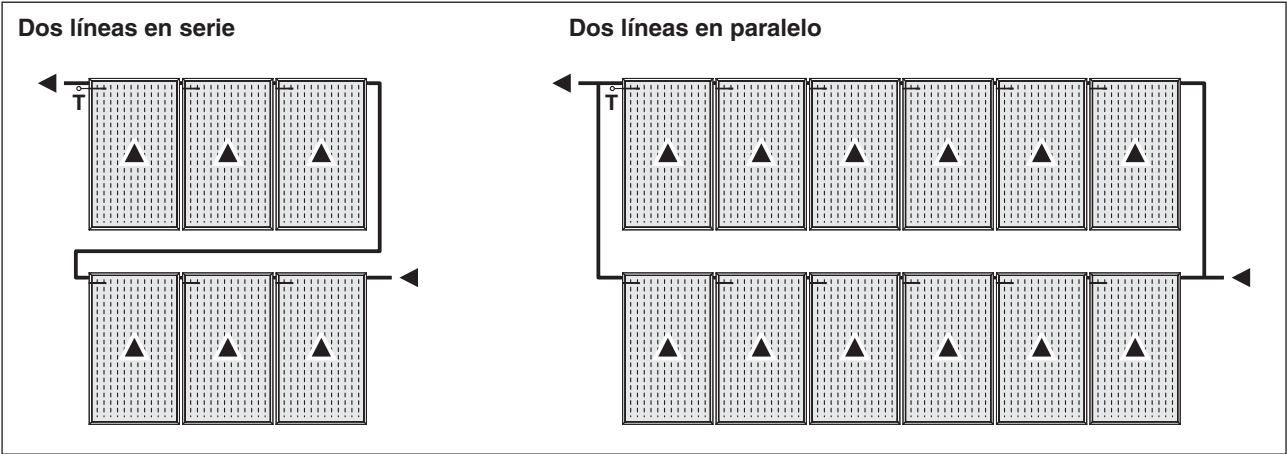
Diámetro tubos de acoplamiento con un caudal específico de 30 litros/m²h
