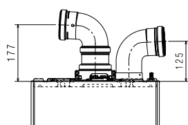
ODVOJENI SISTEM Ø80+80 mm
