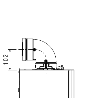
KOAKSIJALNI DIMOVOD Ø60-100 mm
