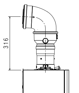
KOAKSIJALNI DIMOVOD Ø80-125 mm
