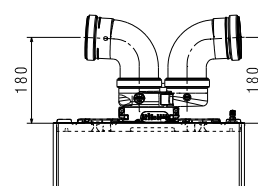
ODVOJENI SISTEM Ø80+80 mm SA KOMPAKTNIM ADAPTEROM
