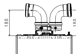
CONDUCTE DIVIZATE Ø80+80 mm CU ADAPTOR COMPACT
