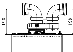
DVOSTRUKI DIMNJAK Ø80+80 mm SA ADAPTEROM
