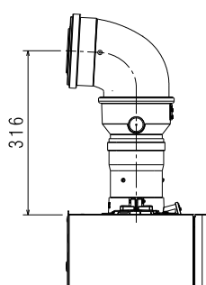
KONCENTRIČNI DIMOVOD Ø80-125 mm
