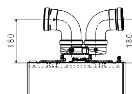
DVOSTRUKI DIMNJAK Ø80+80 mm S KOMPAKTNIM ADAPTEROM
