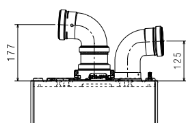
DVOSTRUKI DIMNJAK Ø80+80 mm
