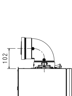
KONCENTRIČNI DIMOVOD Ø60-100 mm
