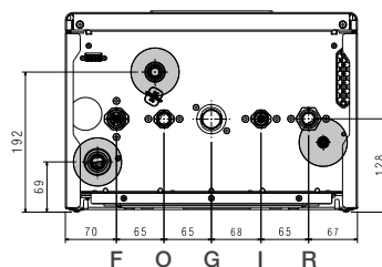
DIN HIDRAULIČKI PRIKLJUČCI
