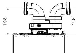
CONDUITE DIVIZATE Ø80-80 mm CU ADAPTOR
