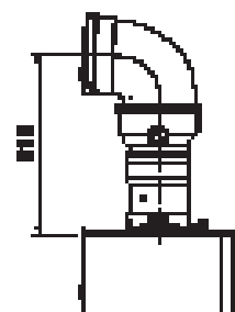
CONCÉNTRICO Ø80-125 mm
