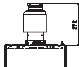
B23P-B53P
