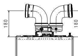
DOBLE CONDUCTO Ø80-80 mm CON ADAPTADOR COMPACTO
