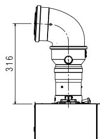
CONDUCTO DE HUMOS CONCÉNTRICO Ø80-125 mm
