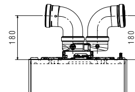
DOBLE CONDUCTO Ø80-80 mm CON ADAPTADOR COMPACTO
