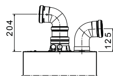
DOBLE CONDUCTO Ø80-80
