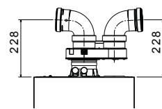
CONDUCTO DOBLE Ø80-80 CON ADAPTADOR
